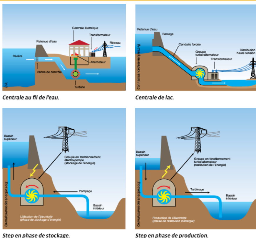
Figure 138 : Schémas des différentes technologies d'ouvrages hydroélectriques
