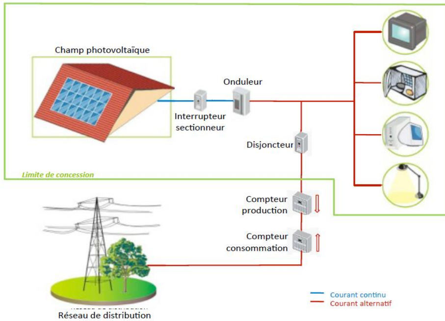
Figure 117 : Fonctionnement d'une installation solaire photovoltaïque en autoconsommation et avec vente de surplus
