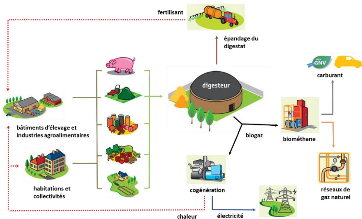
Figure 123 : Schéma de principe du fonctionnement de la méthanisation
