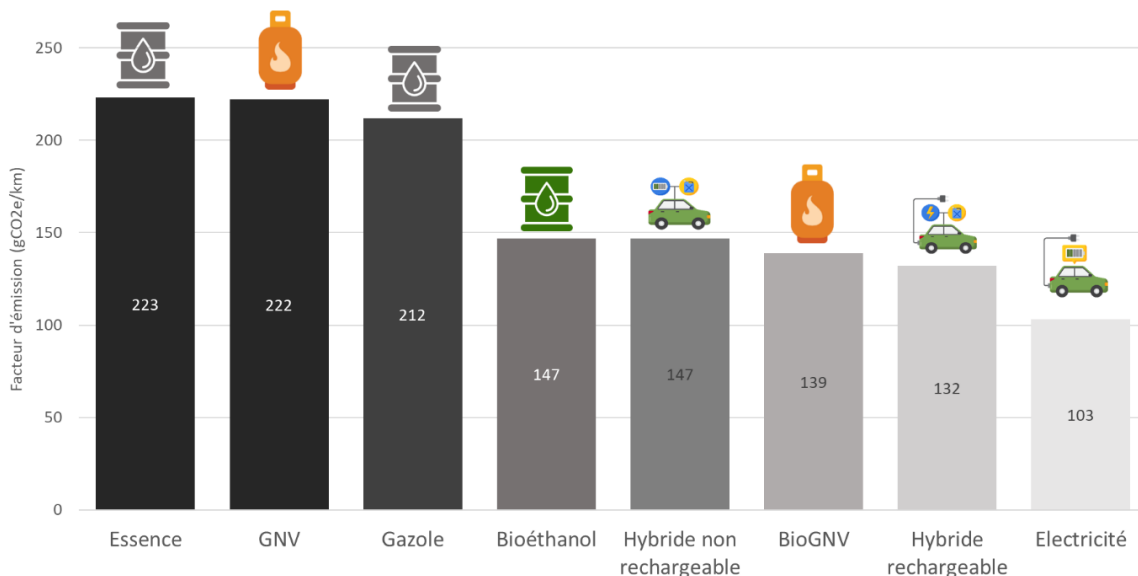
Figure 114 : Facteur d’émission de différentes motorisations, intégrant les émissions liées à la fabrication du véhicule (gCO 2 e/km)
