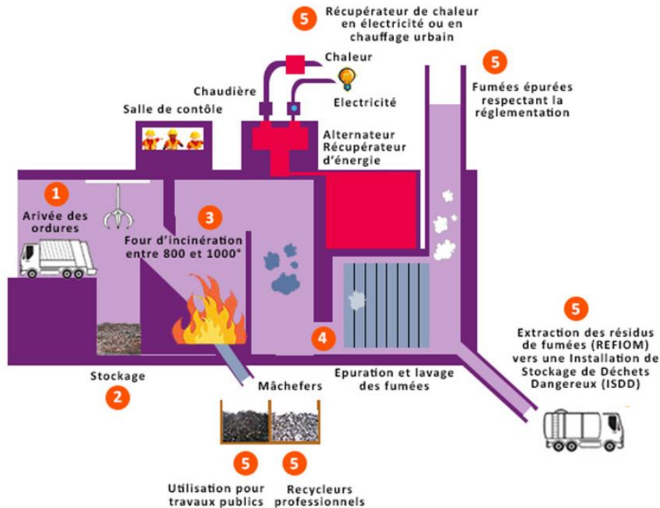
Figure 125 : Schéma d'une unité de valorisation énergétique des déchets
