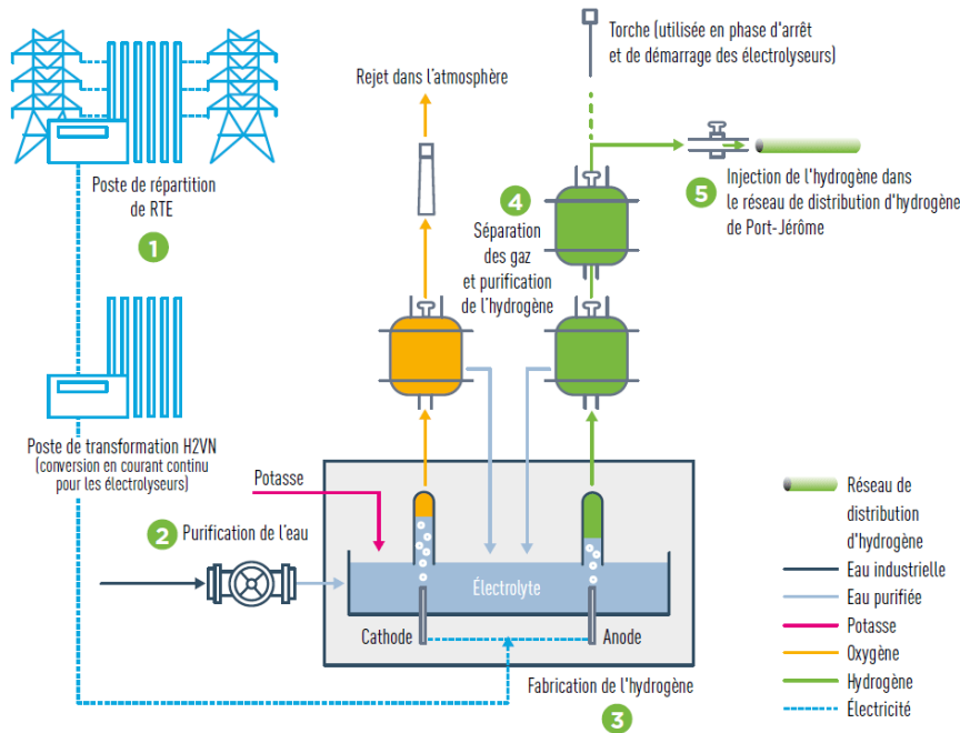
Figure 140 : Production d'hydrogène par électrolyse
