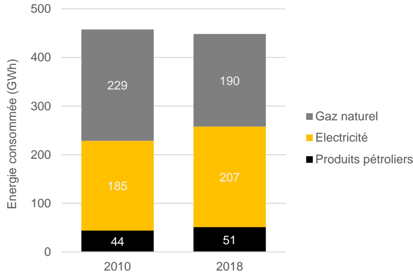
Figure 105 : Consommations d'énergies du secteur Industrie hors branche énergie entre 2010 et 2018
