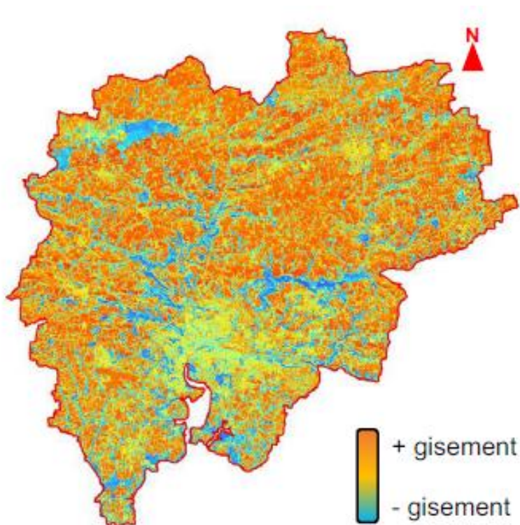
Figure 119 : Carte de gisement solaire sur le territoire de Quimper Bretagne Occidentale
