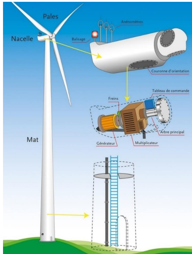
Figure 137 : Fonctionnement d'une éolienne Source : Journal de l'éolien M-A, Guichard Obersy'ER
