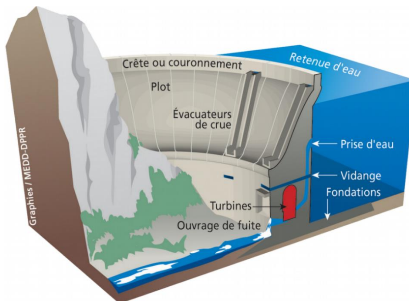
Figure 26 : Constitution d'un barrage voûte
