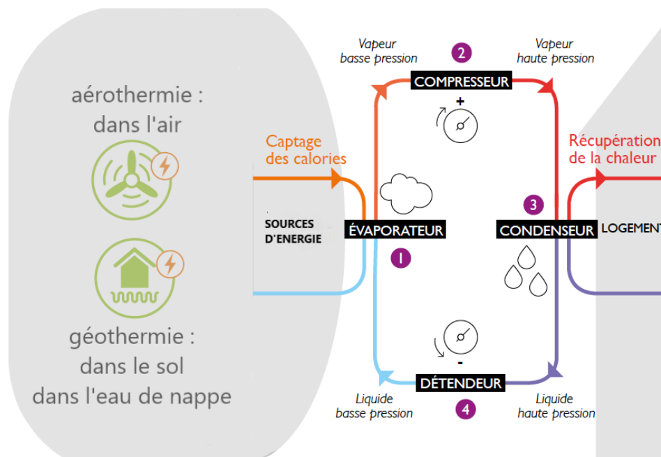
Figure 131 : Schéma de principe de la pompe à chaleur
